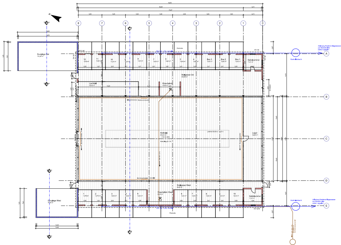
Ebene 0 M 1:100
