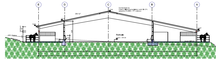
Schnitt 1 M 1:100
